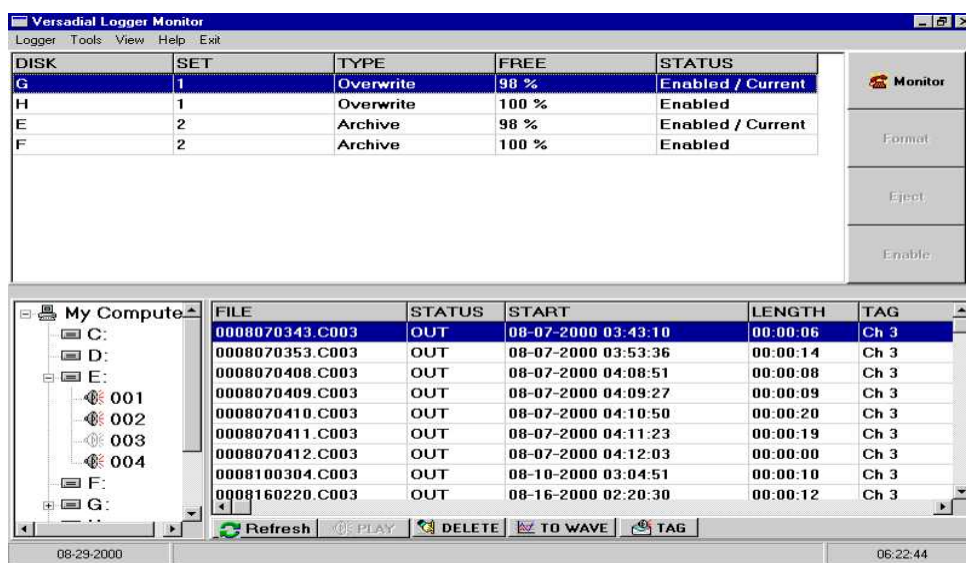
Grafisk brugergrænseflade til styring af Voice-logging
